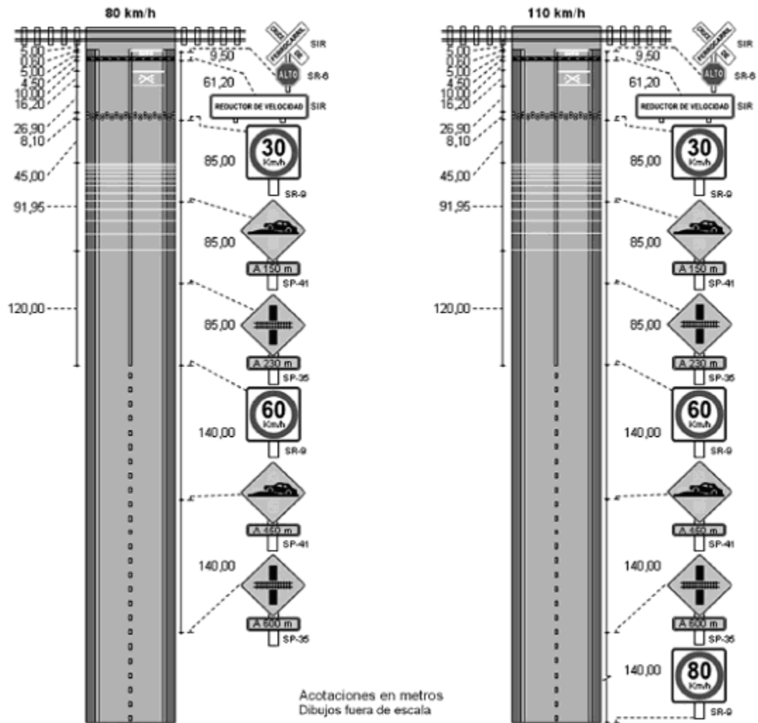
FIGURA B9.- Sistemas de control de velocidad para cruces a nivel con vías de ferreas, cuando las velocidades de operación o de proyecto sean de 80 y 110 km/h
